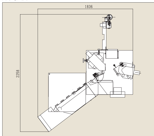
外形寸法図
