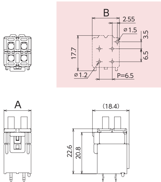
ストレートタイプ (デュアル)
